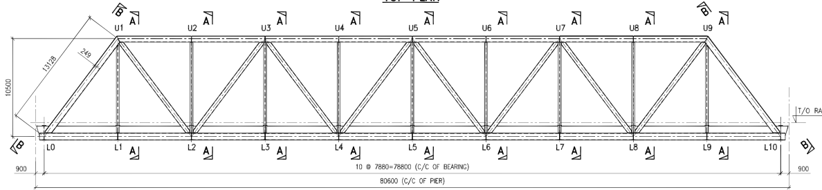
ELEVATION
